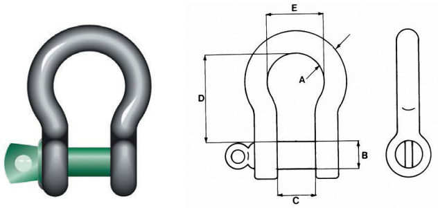
GRILLETE ALTA RESISTENCIA CON CABEZA PASADOR
